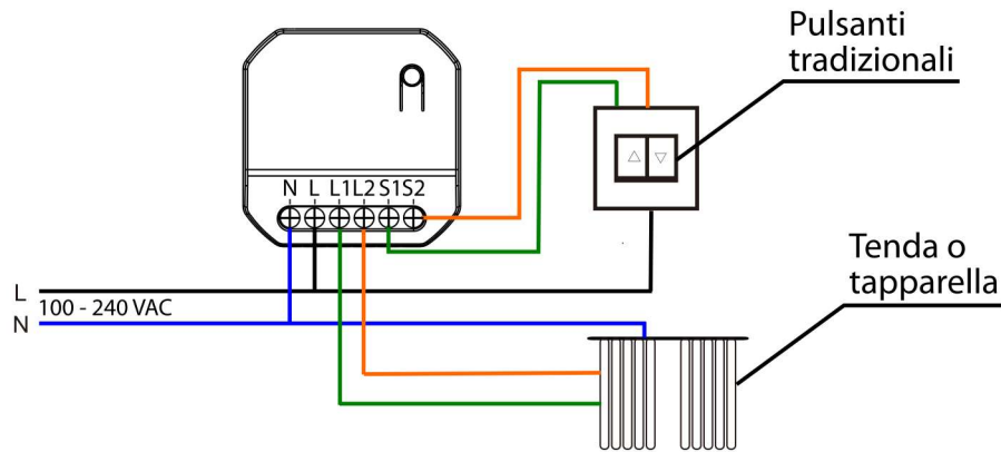
Lo schema di collegamento del 9322
