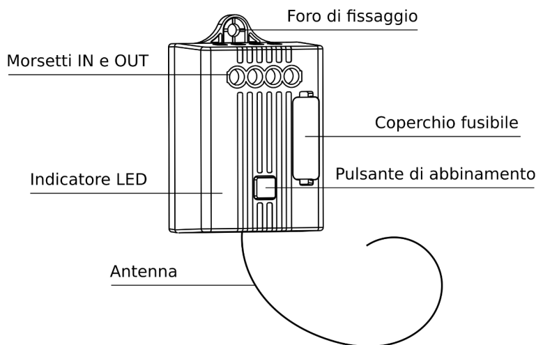
Il vostro Attuatore Smart Wi-Fi 9324
