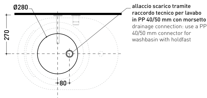
vista pavimento / floor view
