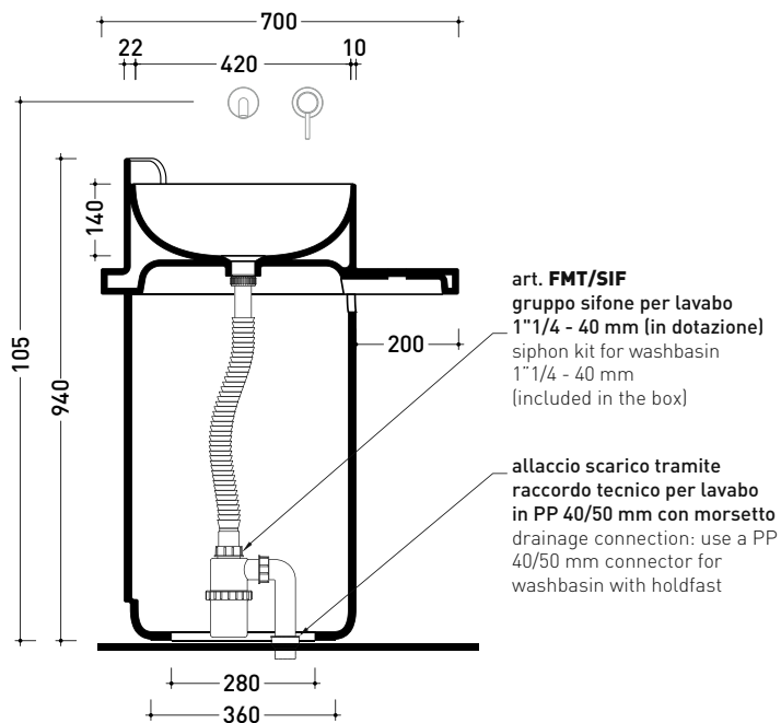
sezione longitudinale / section
