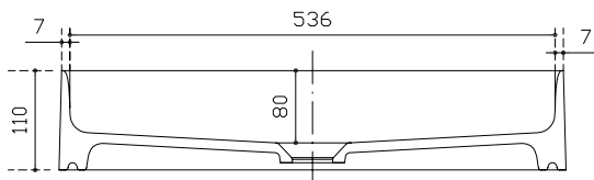
Sezione A-A Section A-A Sección A-A Section A-A
