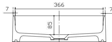
Sezione B-B Section B-B Sección B-B Section B-B
