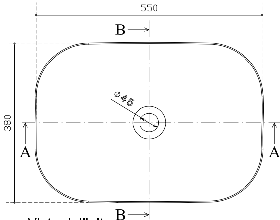
Vista dall'alto View from above Vista desde arriba Vue de dessus
