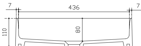
Sezione A-A Section A-A Sección A-A Section A-A
