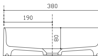
Sezione B-B Section B-B Sección B-B Section B-B
