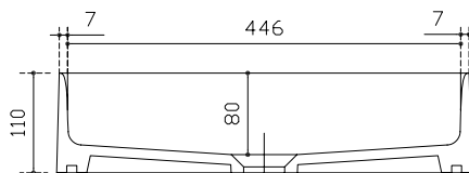
Sezione A-A Section A-A Sección A-A Section A-A
