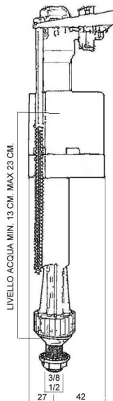
Art. 82 - Alimentazione bassa 3/8 3/8 Bottom float
